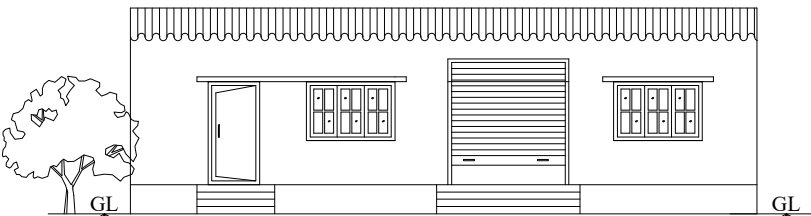
ELEVATION
