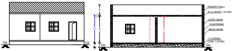
ELEVATION
