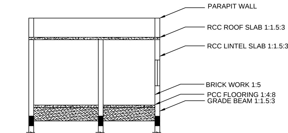
SECTION - AB
