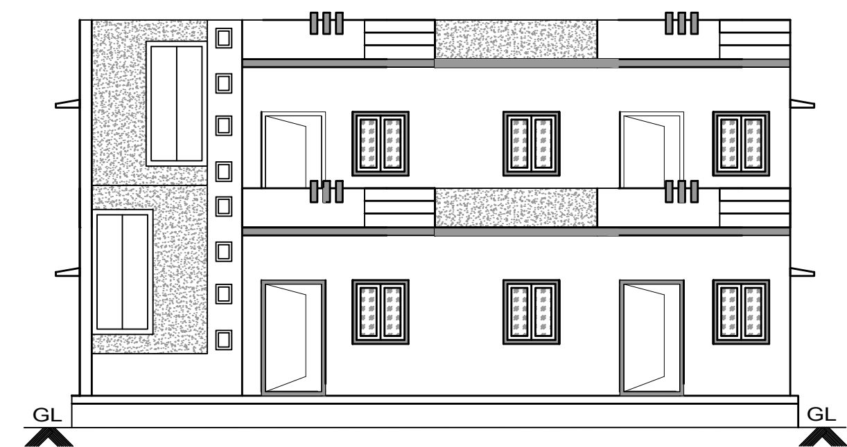
ELEVATION-A
