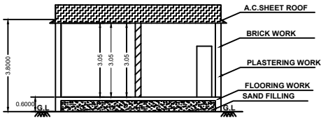
SECTION -AB
