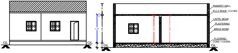
ELEVATION
