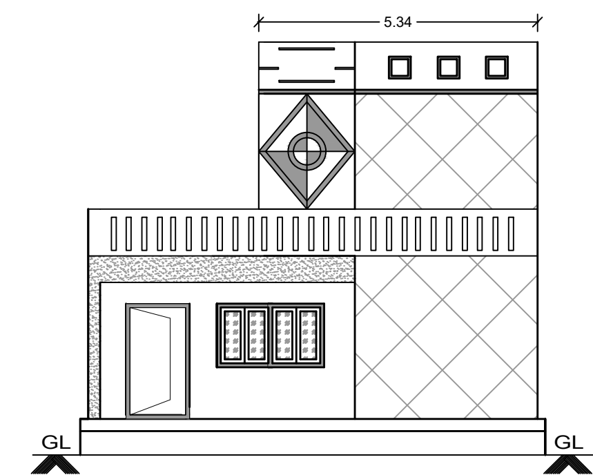
ELEVATION-A
