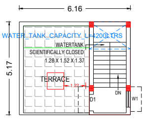
PRO. TERRACE PLAN.
