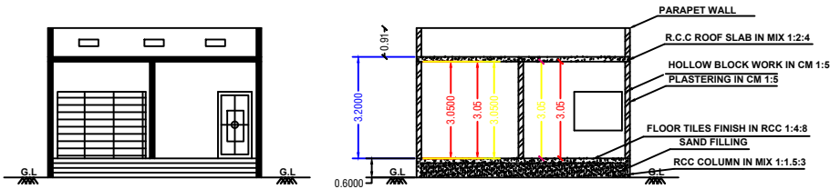
ELEVATION
