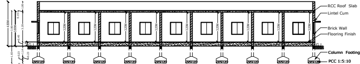
SECTION A-A
