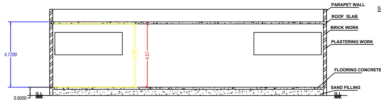
SECTION -AB
