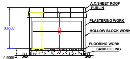
SECTION -AB
