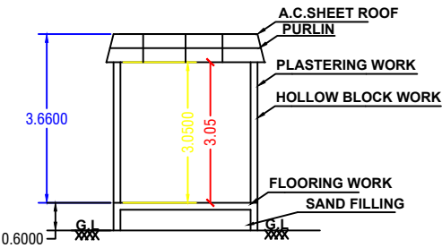
SECTION -AB
