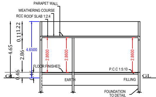
SECTION - AB
