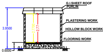
SECTION -AB
