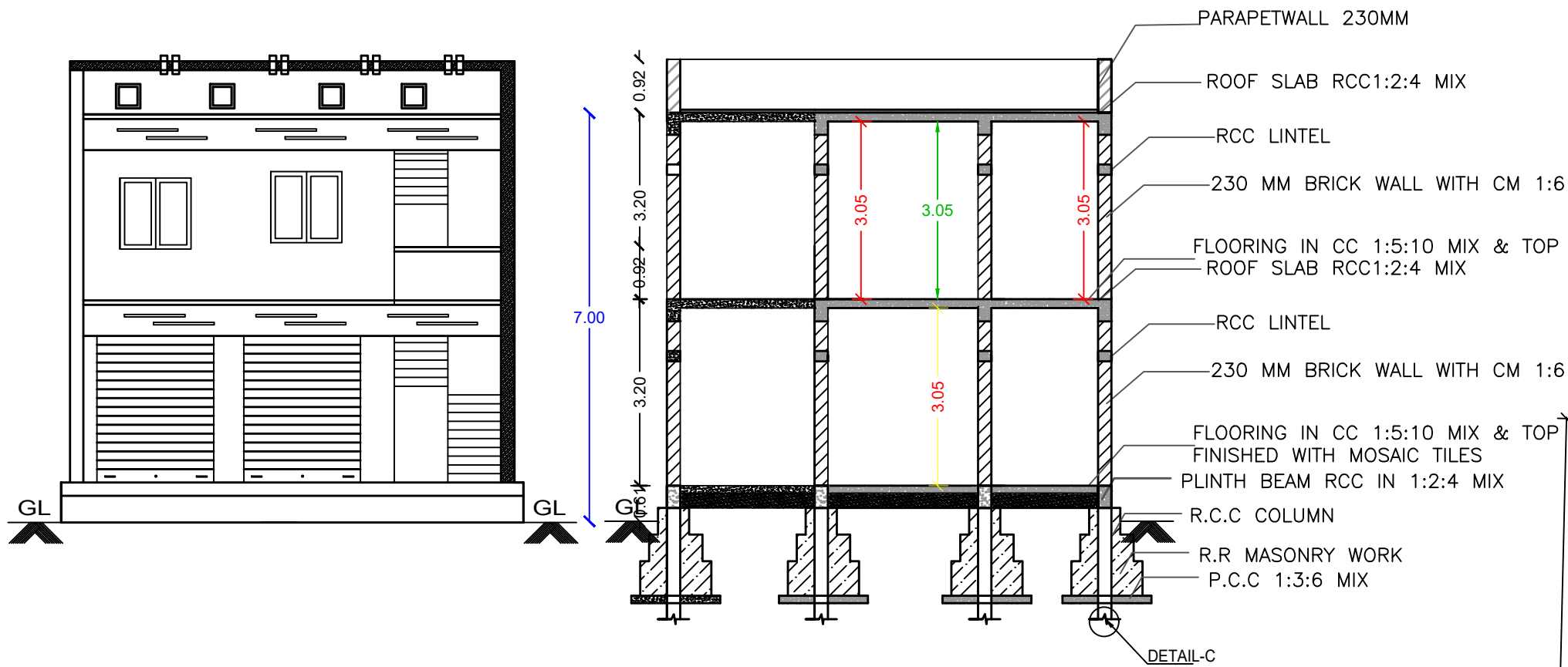
ELEVATION-A
