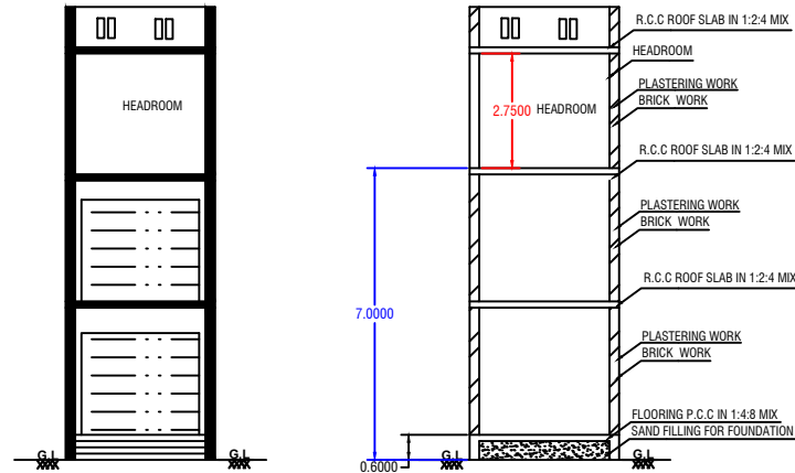
ELEVATION
