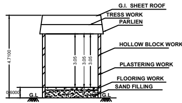
SECTION -AB
