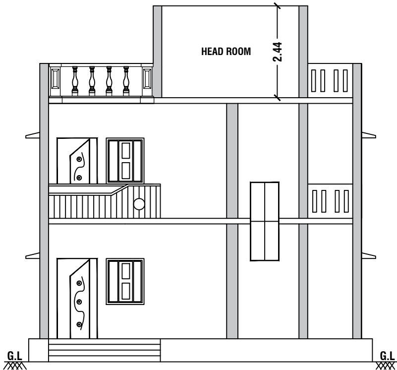
ELEVATION
