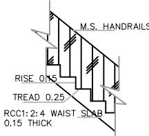
STAIRCASE DETAILS SCALE: 1:20
