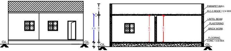
ELEVATION
