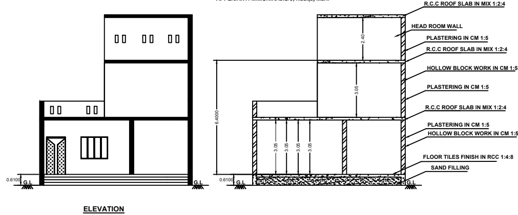
SECTION -AB
