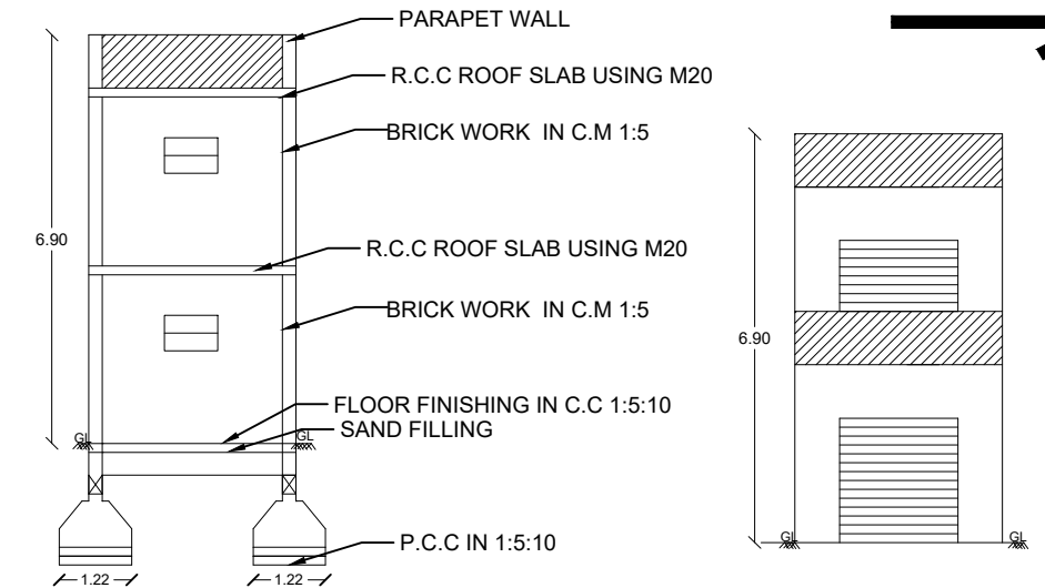
ELEVATION
