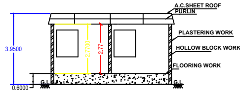
SECTION -AB
