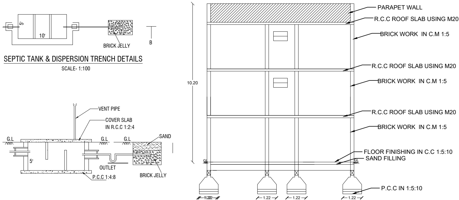
SECTION A-A
