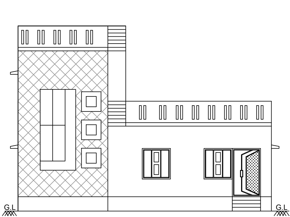
ELEVATION-A
