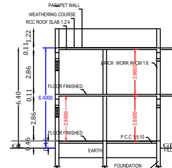
SECTION - AB
