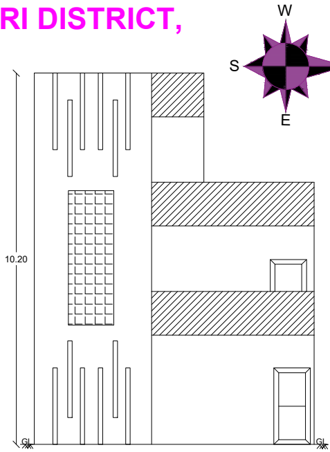
ELEVATION
