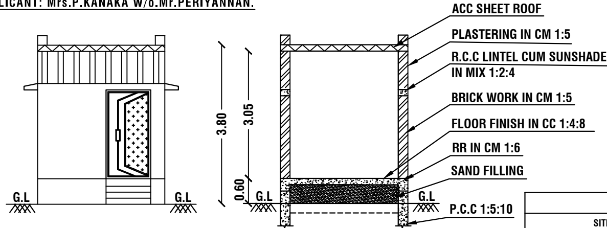
ELEVATION
