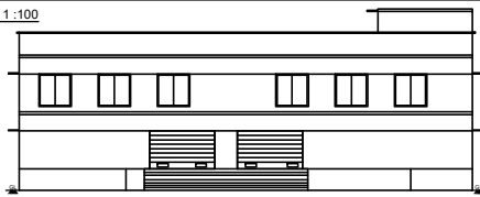
ELEVATION 25.46
