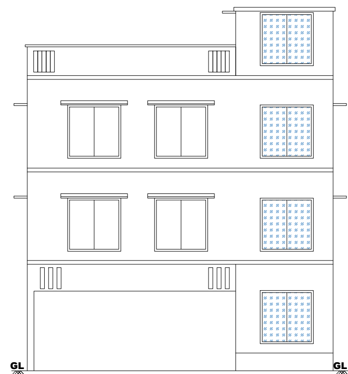
ELEVATION
