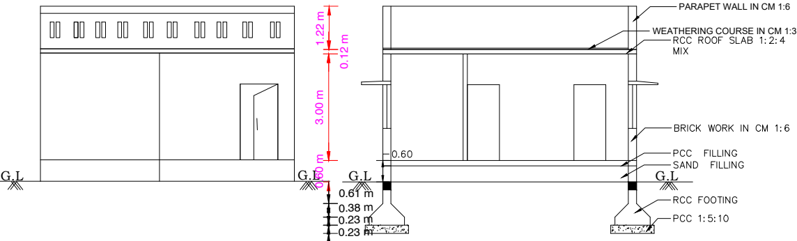
ELEVATION
