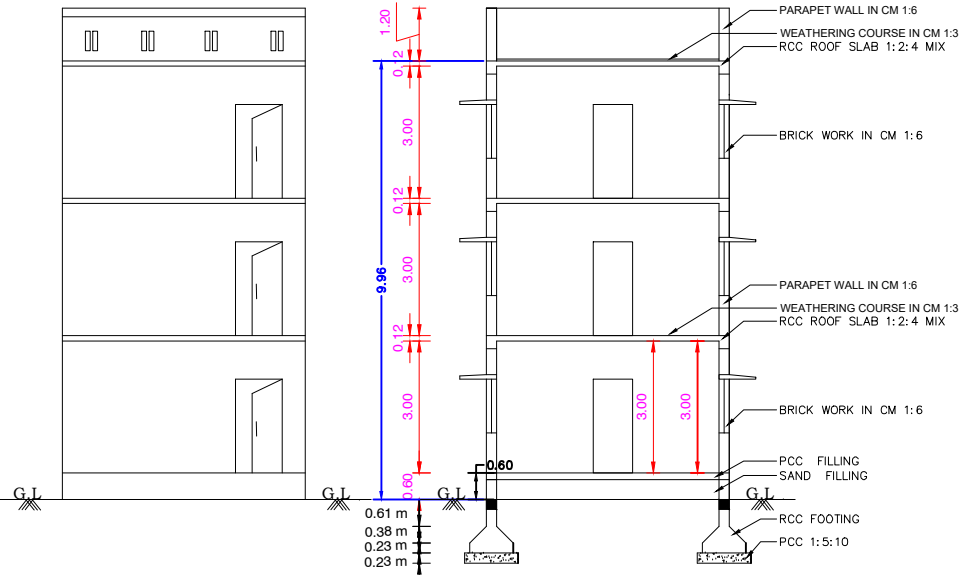
ELEVATION
