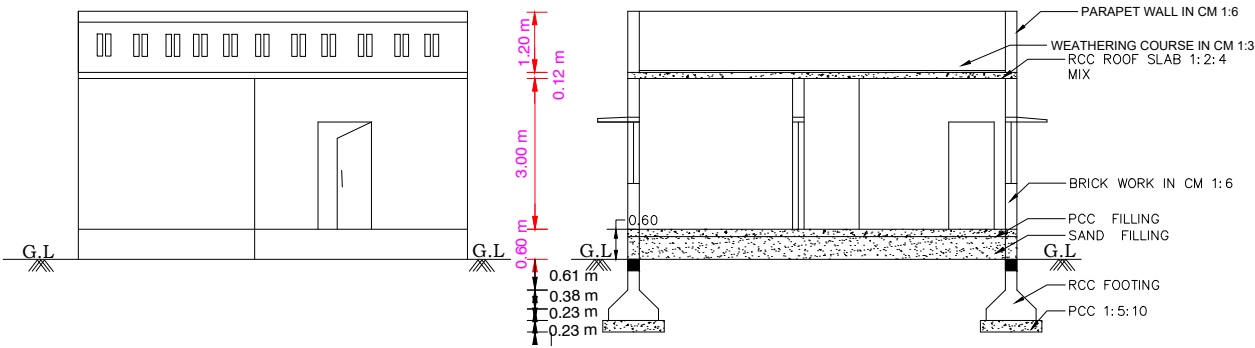
ELEVATION
