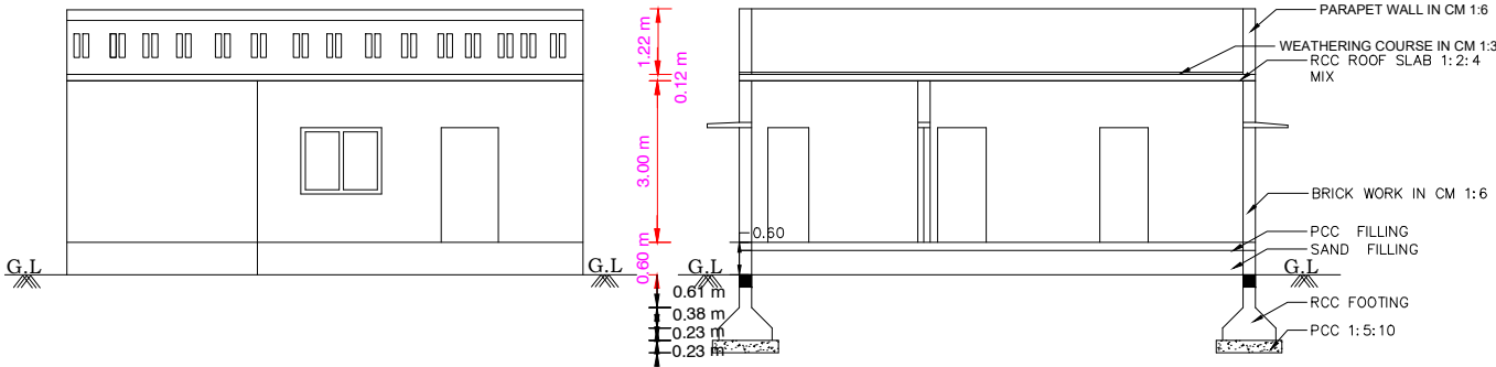
ELEVATION
