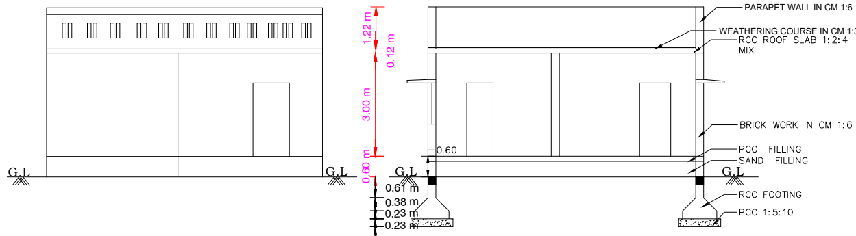
ELEVATION
