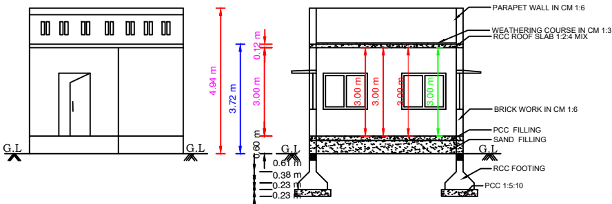
ELEVATION
