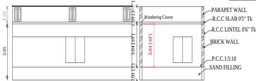
ELEVATION
