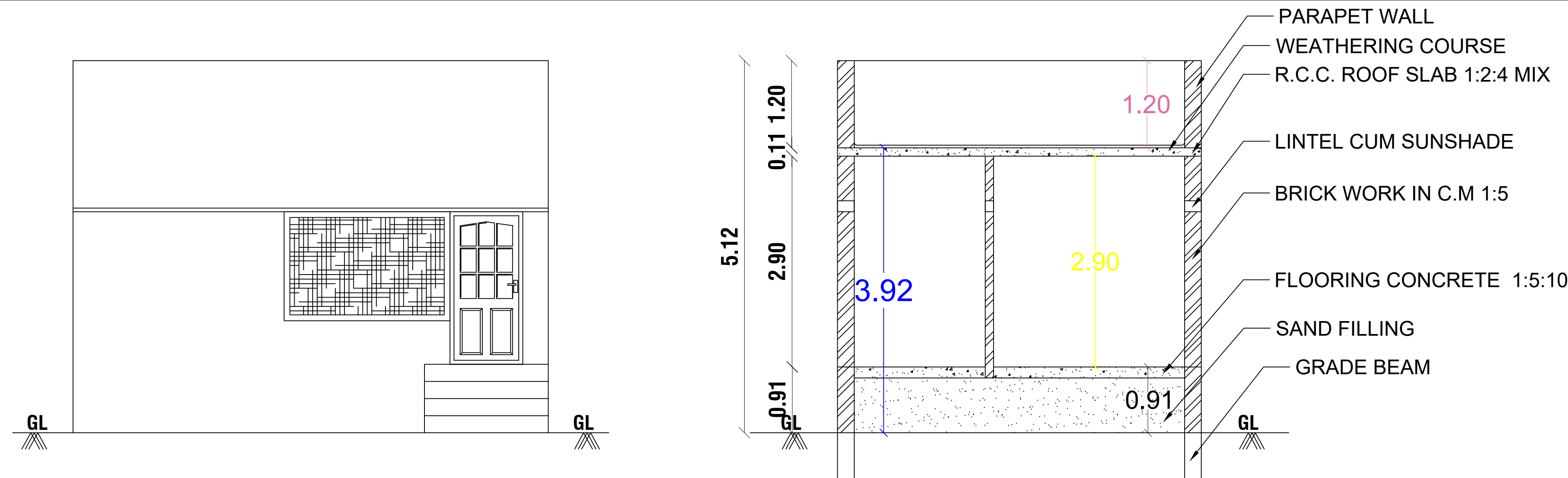
ELEVATION
