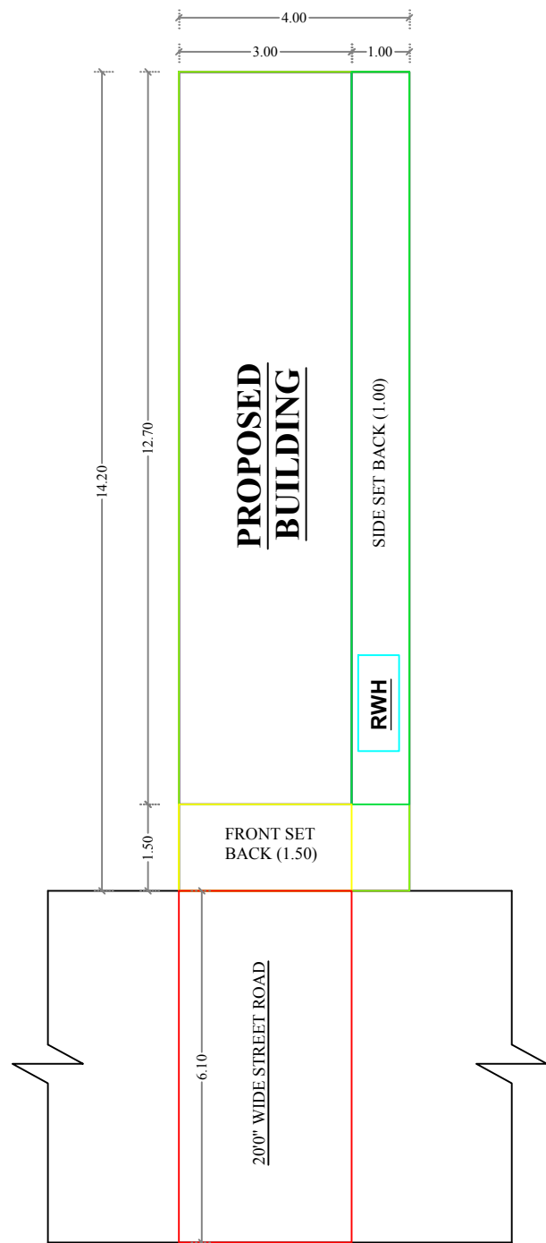
.SITE PLAN.
