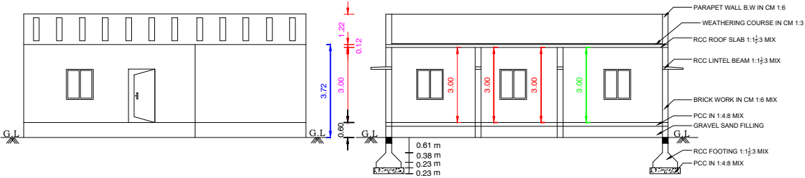
ELEVATION
