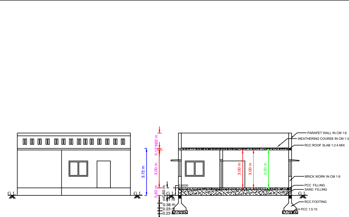
ELEVATION
