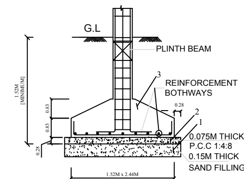
TYP. DET. COLUMN FOOTING
