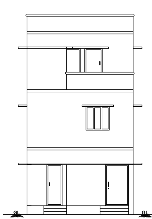
ELEVATION
