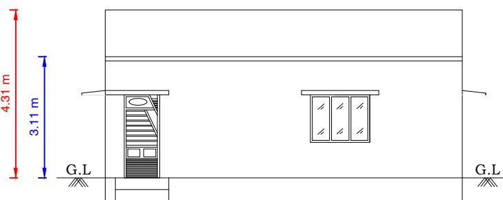
ELEVATION
