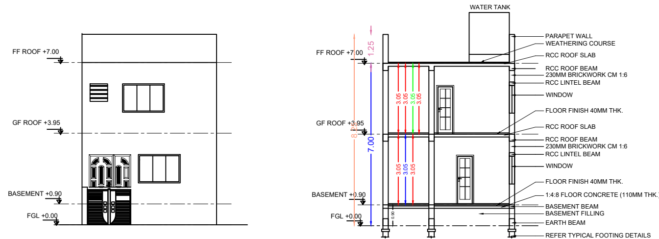
1 ELEVATION
