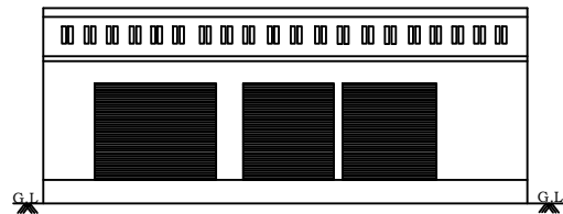
ELEVATION
