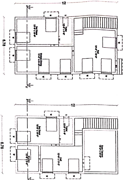
PRO G.F PLAN
