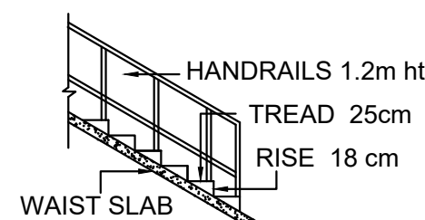
STAIRCASE DETAILS (N.T.S.)
