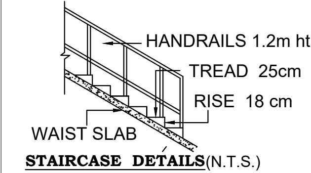
STAIRCASE DETAILS (N.T.S.)
